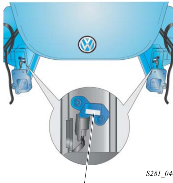
Опережающие датчики удара в лонжеронах кузова
