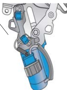
Датчики блокировки верха слева F323 и F324, а также двигатель блокировки слева V291
