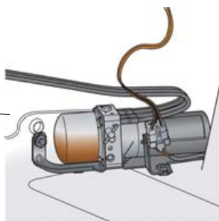
Гидронасос привода складного верха V118
