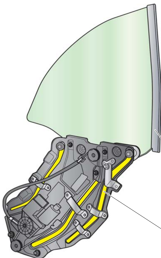
Направляющая стекла
