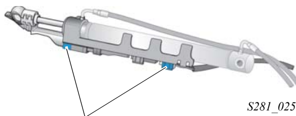
Датчики F171
