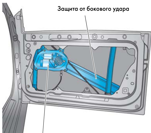
Двигатель стеклоподъемника
